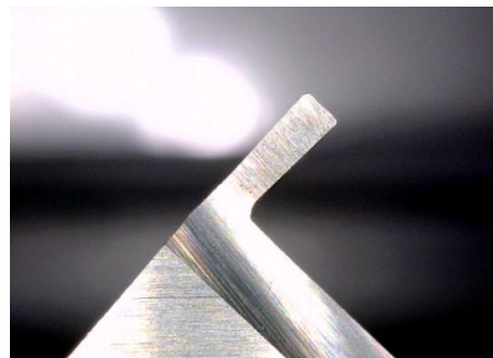
超硬溝入れバイト製作 0.2t × 0.35 × φ4 (展示品6)
