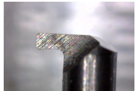
超硬溝入れバイト製作0.7t (展示品6)
